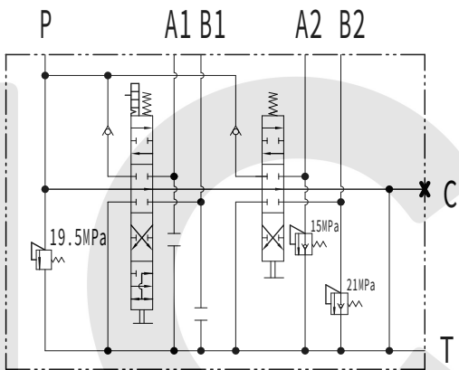
液压原理图
