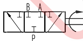
O型原理图
