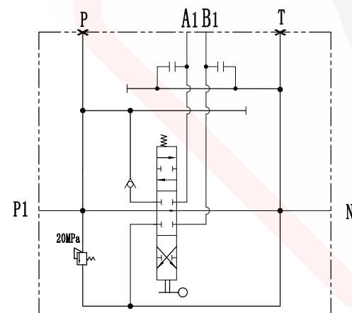
液压原理图
