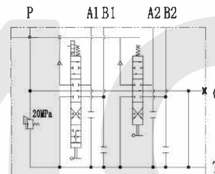
液压原理图
